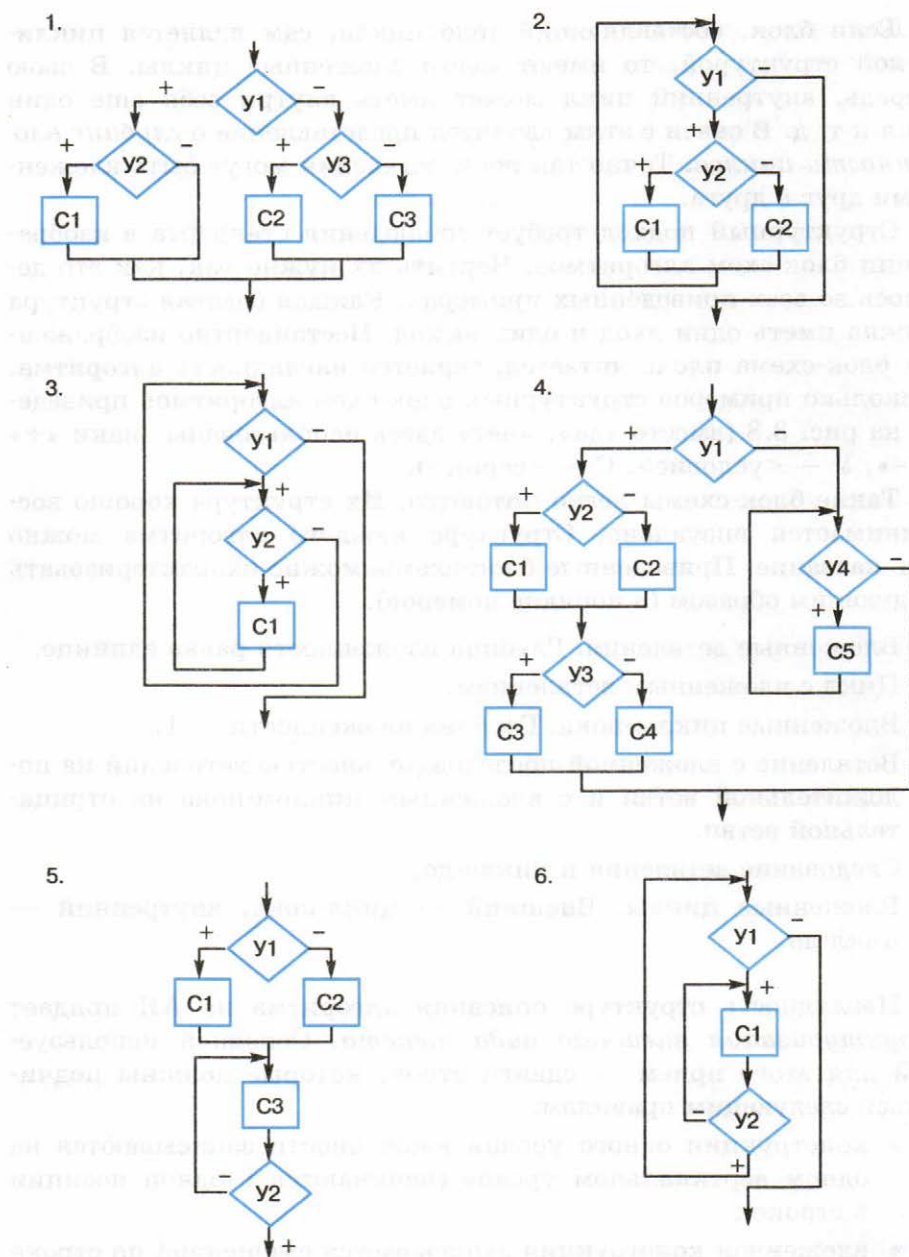
Рис. 3.8. Структурные схемы алгоритмов
