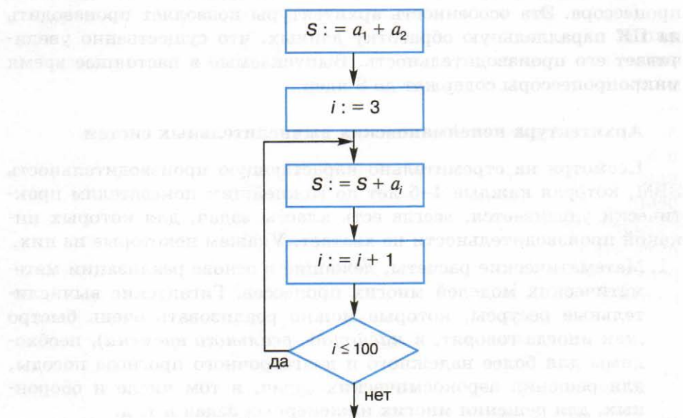
Рис. 2.8. Алгоритм решения задачи последовательного сложения массива чисел
