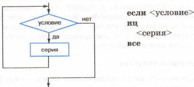
Рис. 3.6. Структура «цикл-пока»
