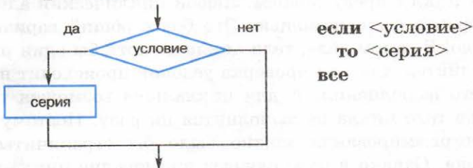
Рис. 3.5. Неполное ветвление
